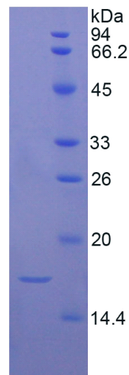
15% SDS-PAGE
