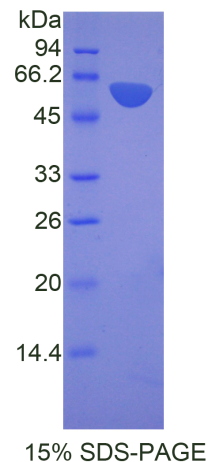
15% SDS-PAGE
